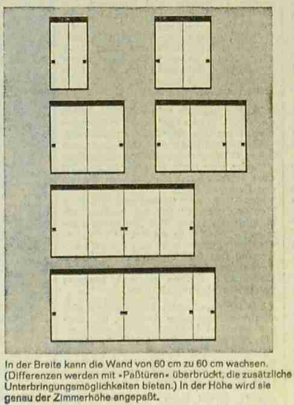
In der Breite kann die Wand von 60 cm zu 60 cm wachsen. (Differenzen werden mit „Puffüren“ überbrückt, die zusätzliche Unterbringungsmöglichkeiten bieten.)
